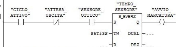
Segmento 5 : Allo scadere del tempo eseguo la marcatura
