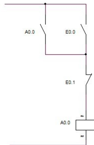
Segmento 1 : Set dell'uscita
