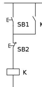
Fig.1.a. schema funzionale
