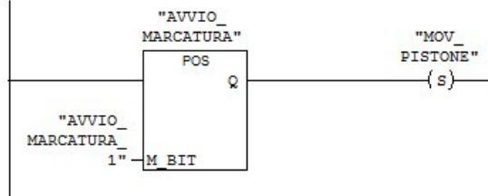
Segmento 6 : Dopo 5 secondi che il pistone va in basso spengo il movimento
