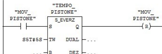
Segmento 6 : Dopo 5 secondi che il pistone va in basso spengo il movimento
